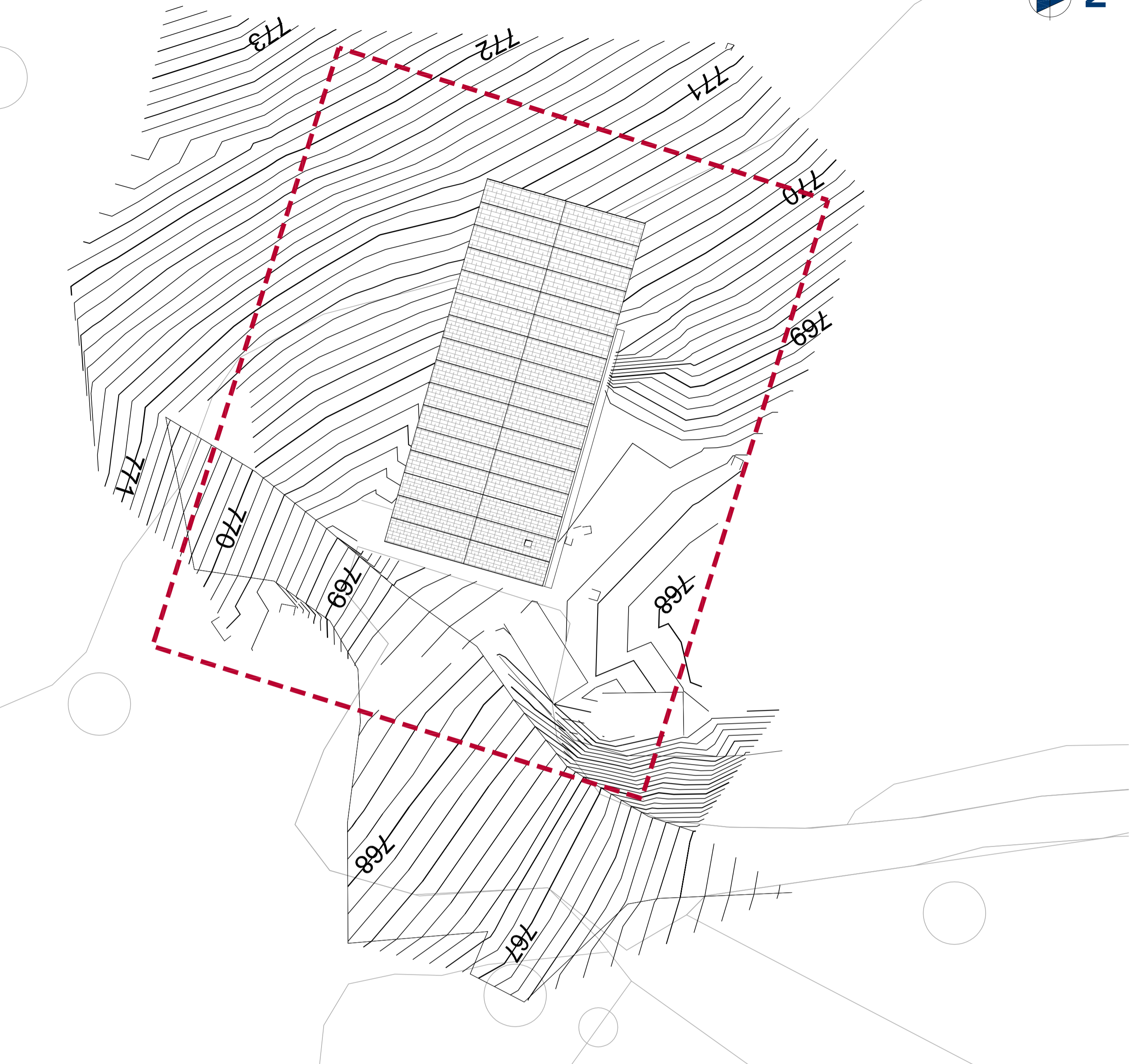
Planimetria di progetto - scala 1:200
